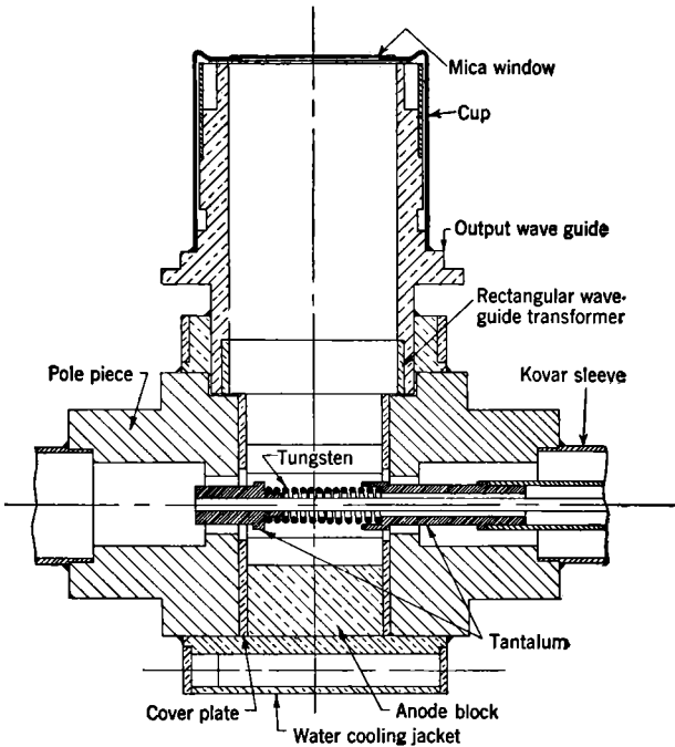
FIG. 19-69.—Longitudinal cross section of XCR magnetron.
